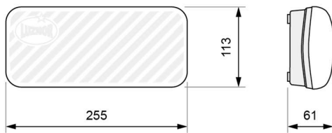
Montaje en superficie
