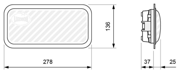
Montaje empotrado (corte: 265 x 120 mm)
